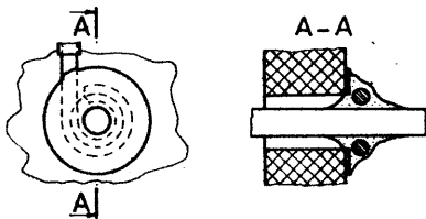
Obr. 10. Vodič ve tvaru oka na osazeném pájecím bodě. Očko nesmí přesahovat pájecí bod. Příklad jednovrstvé desky s plošnými spoji s neprokovennými otvory
